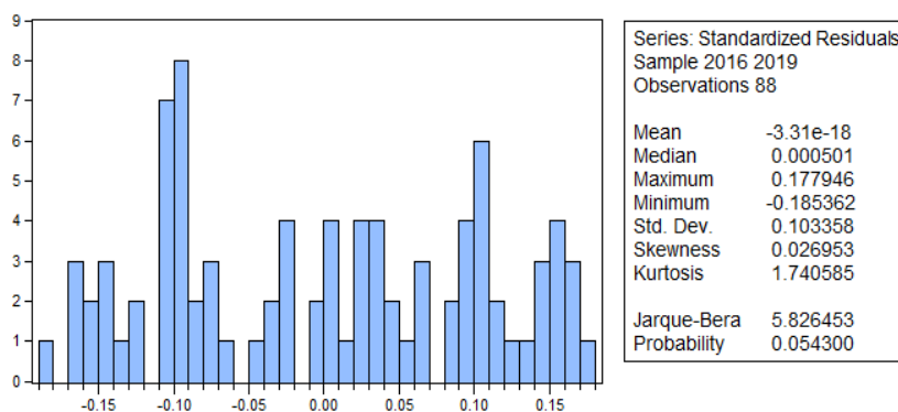
Gambar 1. Uji Normalitas
