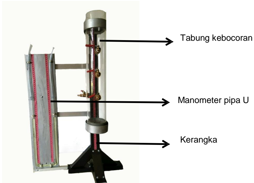
Gambar 1. Alat peraga tekanan hidrostatik
