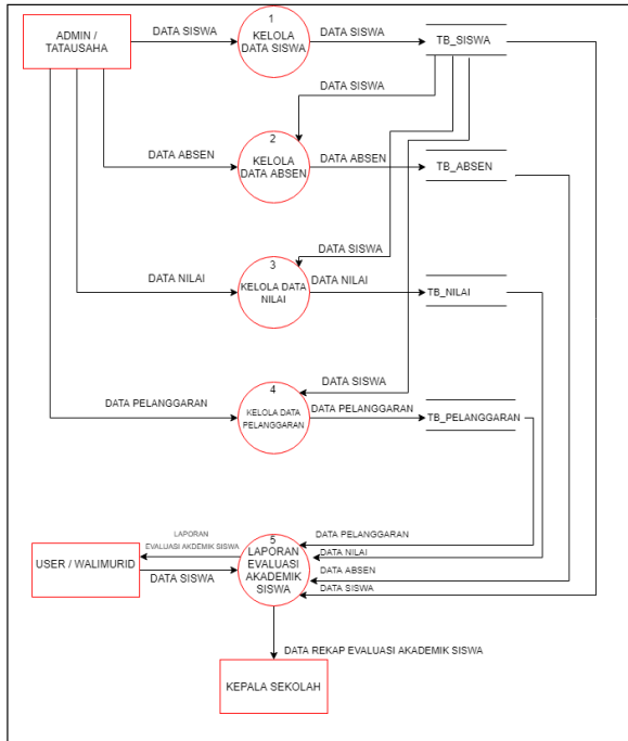
Data Flow Diagram (DFD) level satu yang diusulkan
